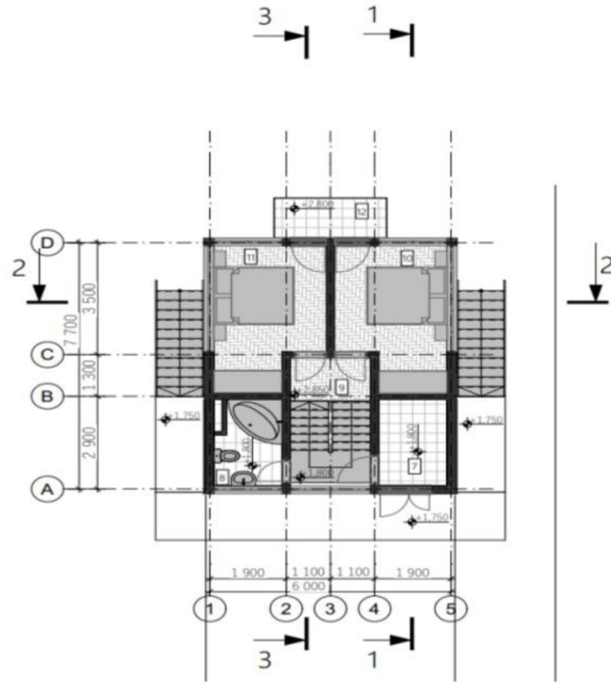
Plan Etaj amenajare , cota +2,800, sc. 1:100
