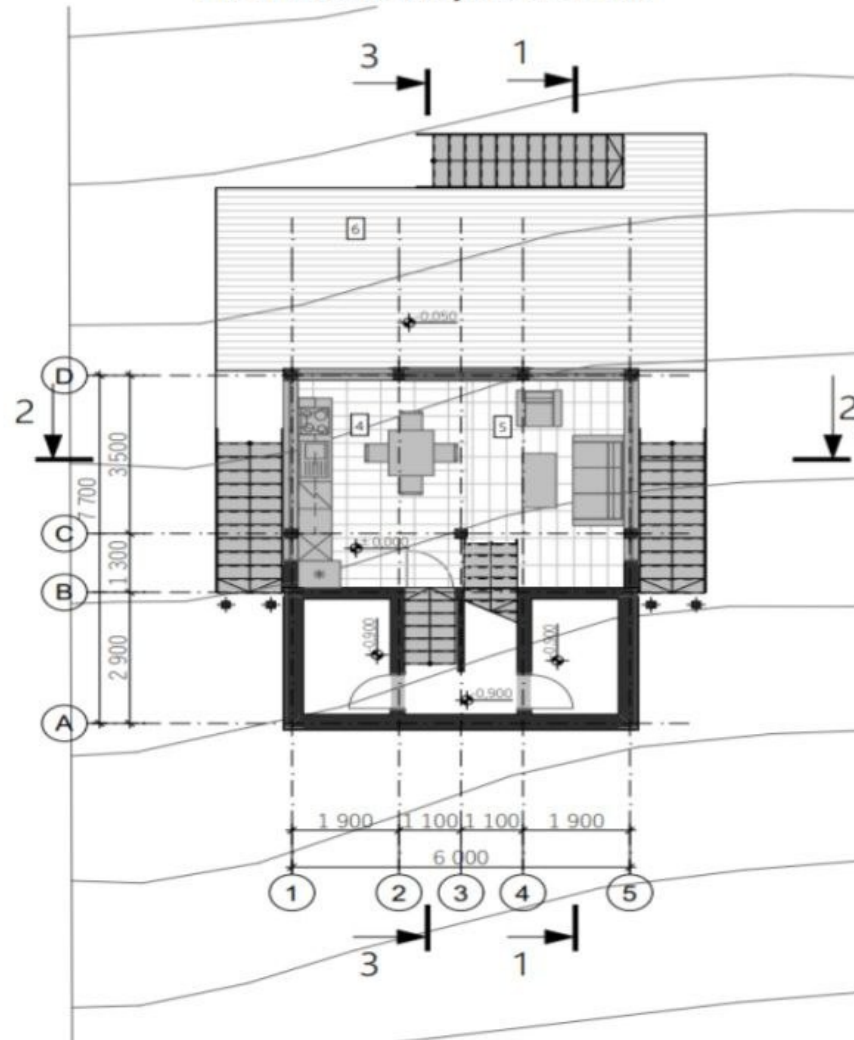
Plan Parter amenajare, sc. 1:100
