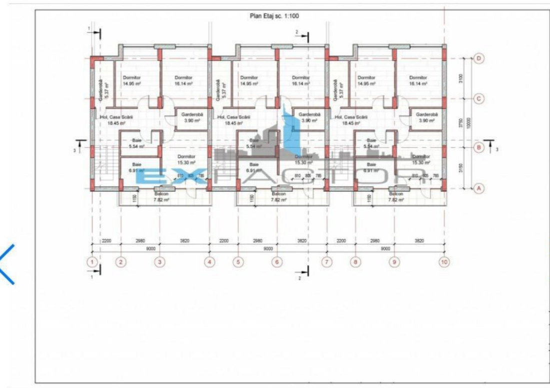
Plan Etaj 300.00 m.p.
