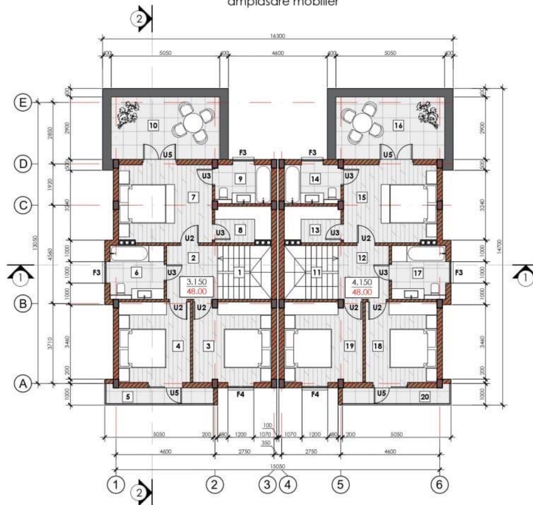
Plan etaj, sc. 1:100, amplasare mobilier
